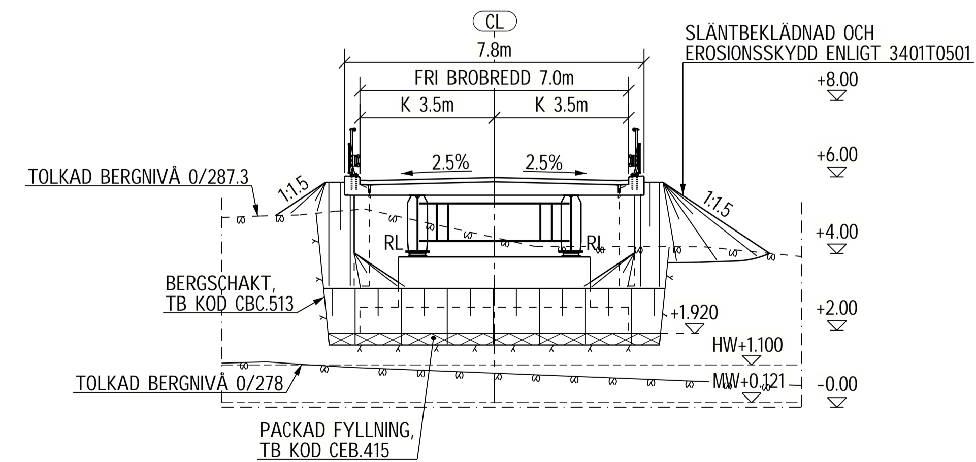
SEKTION C - C 1:100 3441K2001
