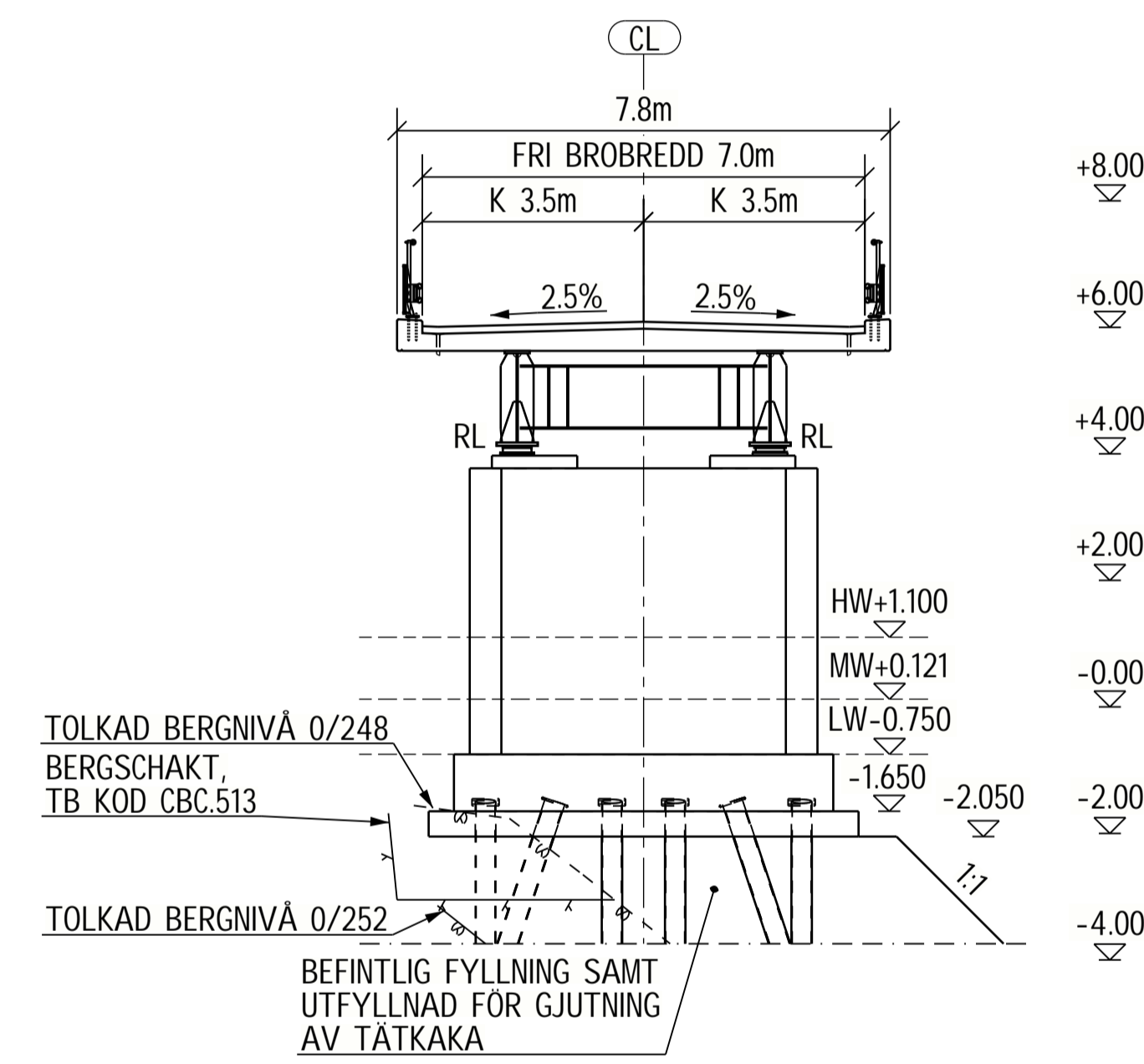
SEKTION B - B 1:100 3441K2001
